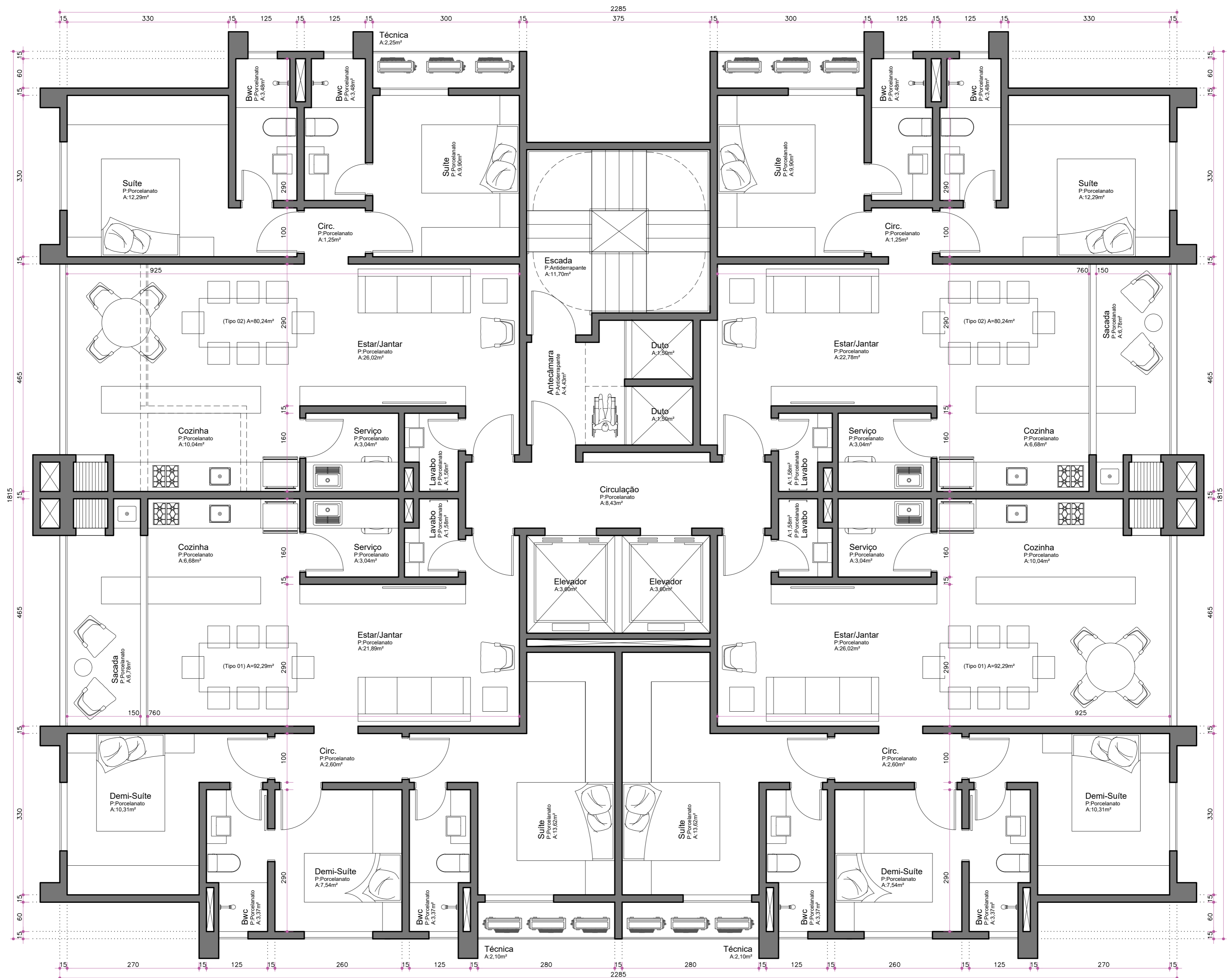
Planta Baixa Pavimento Tipo (x9)
